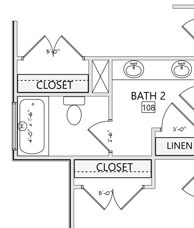
OPTIONAL BATH 2
